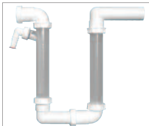
Рис. 2. Сифон HL 136.2
