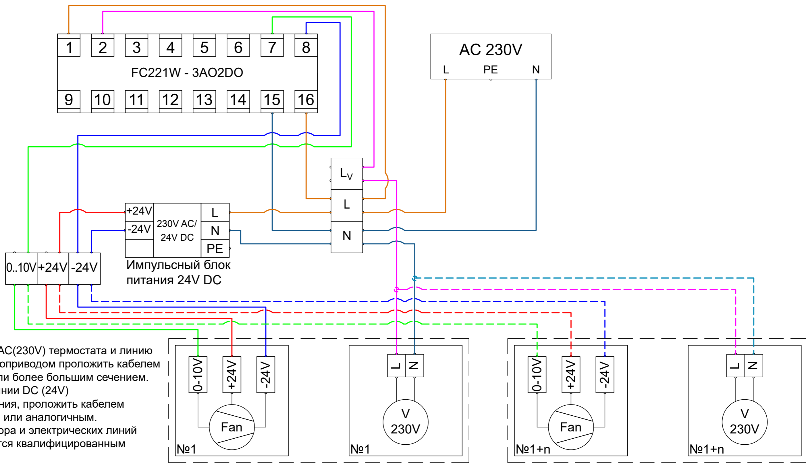
Схема подключения термостата FC221W-3AO2DO с WiFi модулем к внутрипольному конвектору (QSKS/QSKM) - 230V
